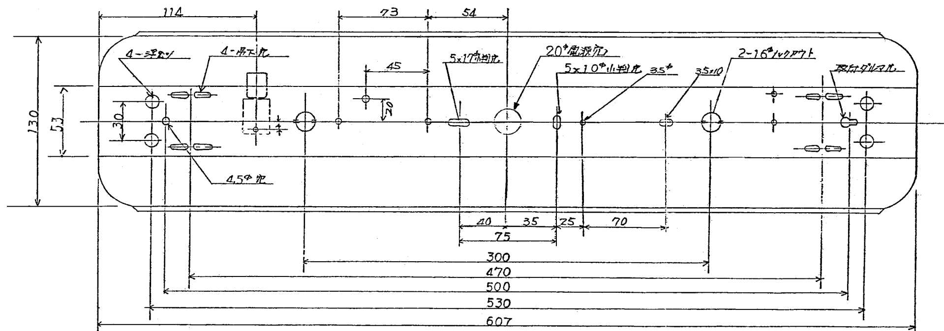
取付背面図 s=1/2
