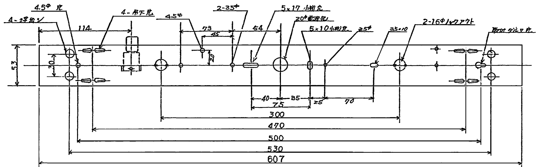
取付背面図5=1/2
