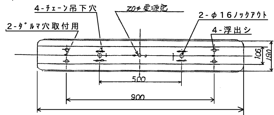
取付背面図 S=1/10
