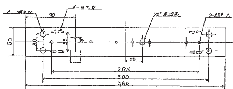
取付背面図 5=1/2
