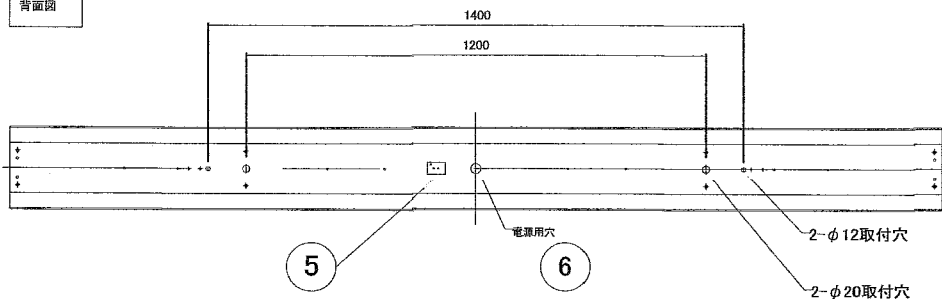
背面図
