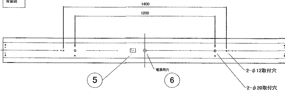
背面図
