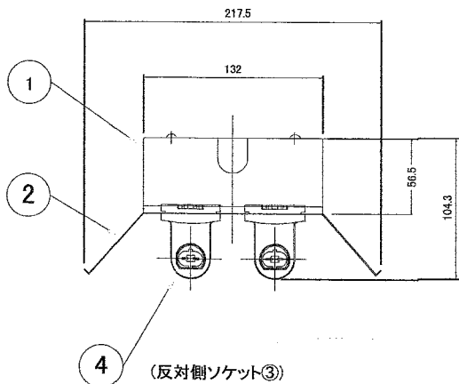
背面図
