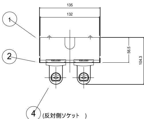
背面図
