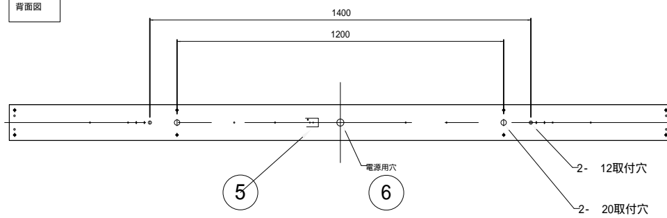
背面図
